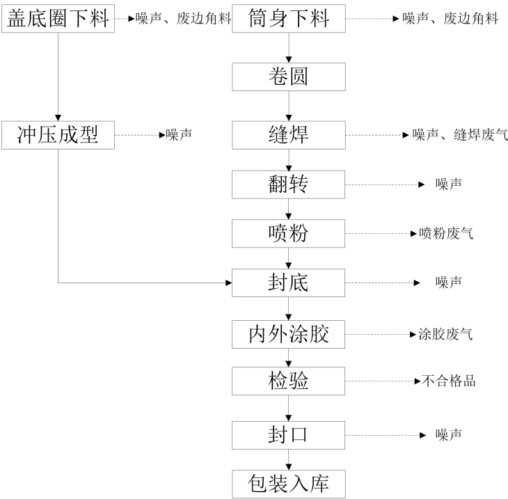
图 3-4 制罐生产工艺流程及产污环节图
