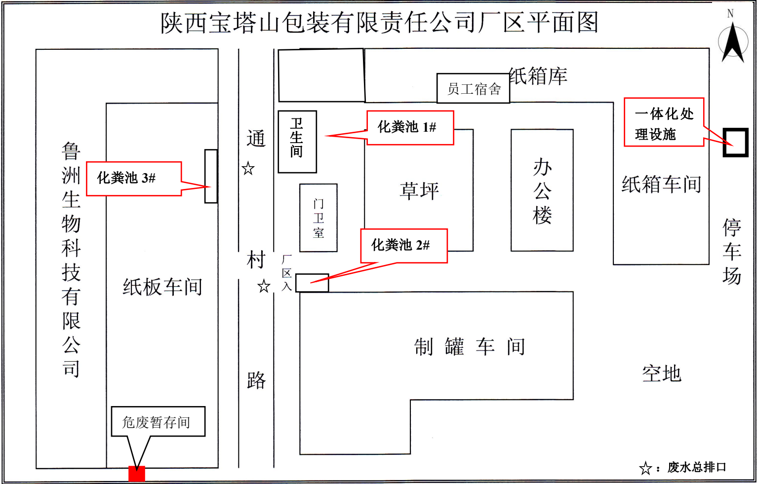
图 3-2 项目厂区平面布置图
